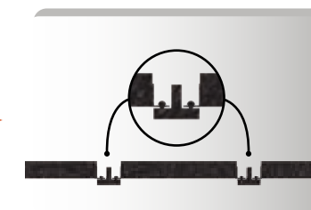
EN JOINTS CREUX SUR SUPPORT EN "T" / OPEN VOEGEN OP "T"-PROFIEL
