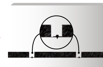
EN JOINTS CREUX SUPERPOSÉS / OVERLAPPENDE OPEN VOEGEN
